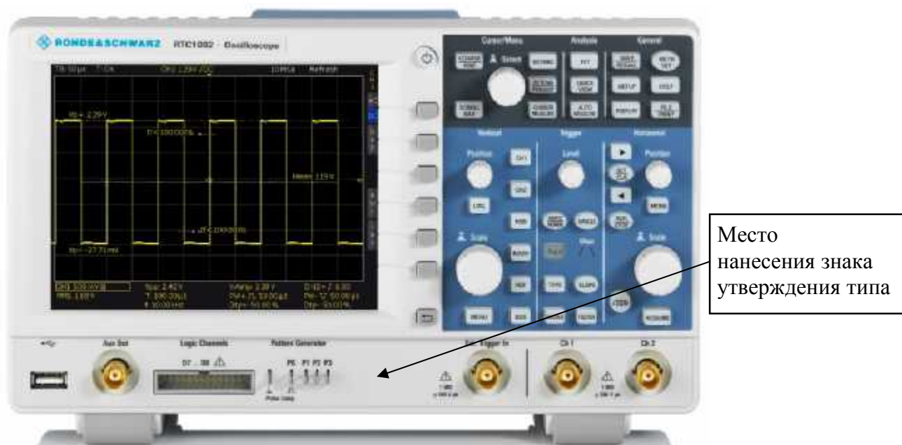
Рисунок 1 - Общий вид средства измерений и обозначение мест нанесения знака утверждения типа
