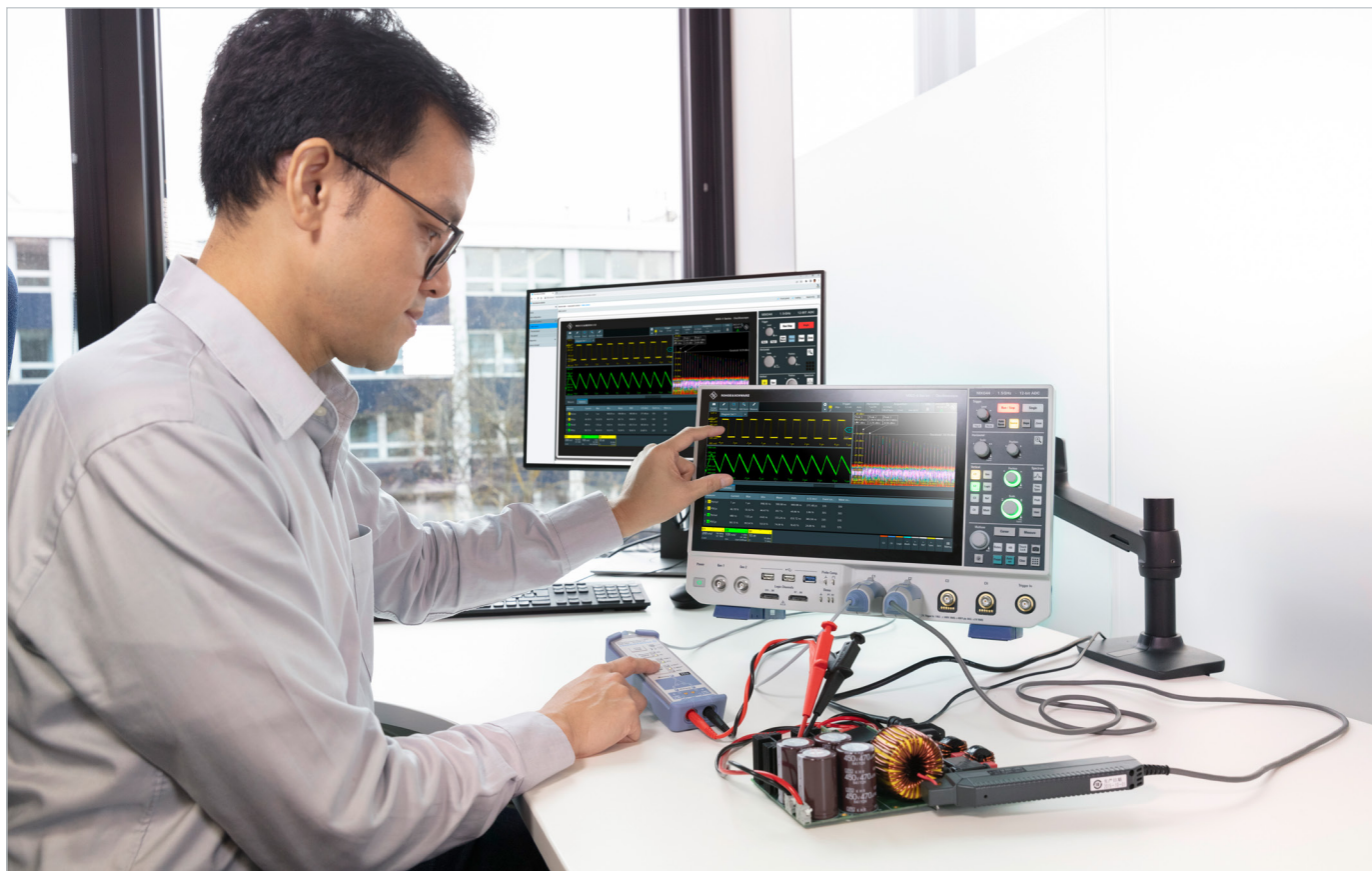
Высоковольтные дифференциальные пробники для анализа мощности переключения.
