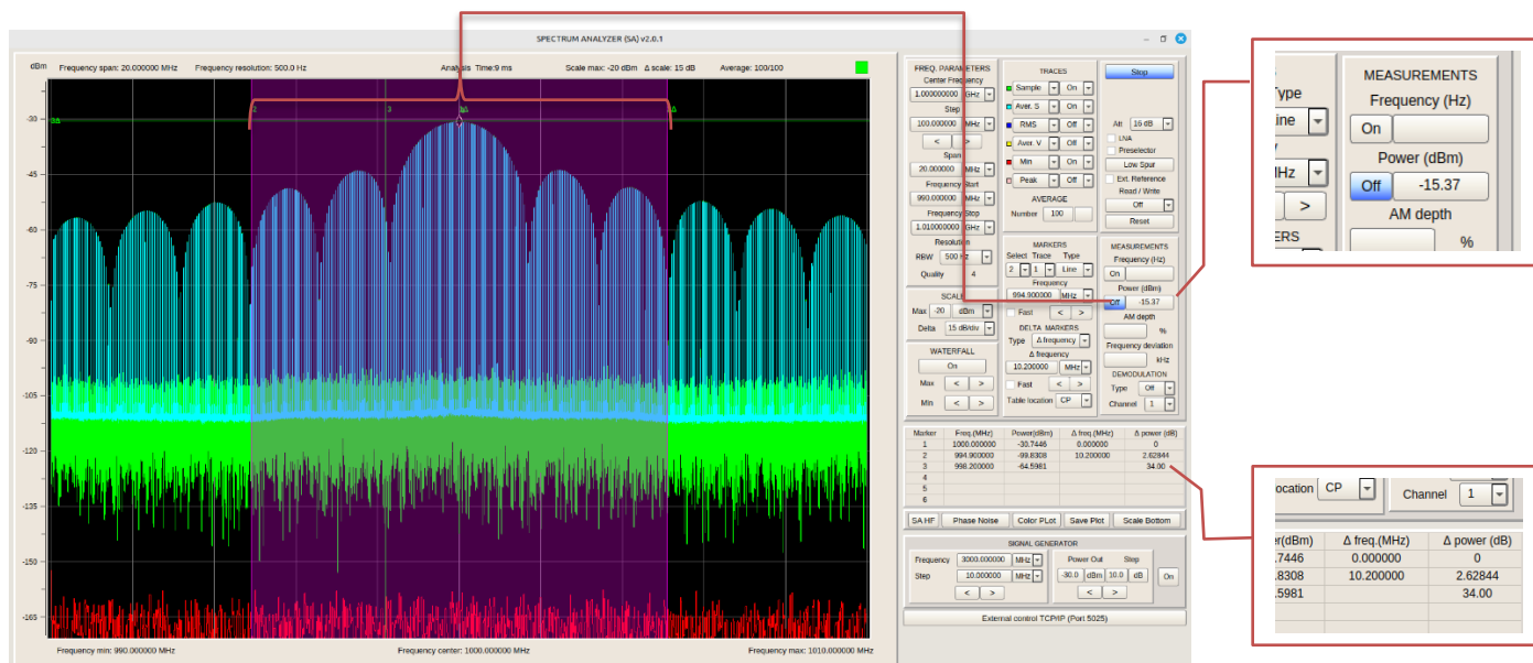
Рис. 2. Режим частотной развертки с применением различных маркеров (измерения дельта-величин и интегральных значений внутри выделенной области)
