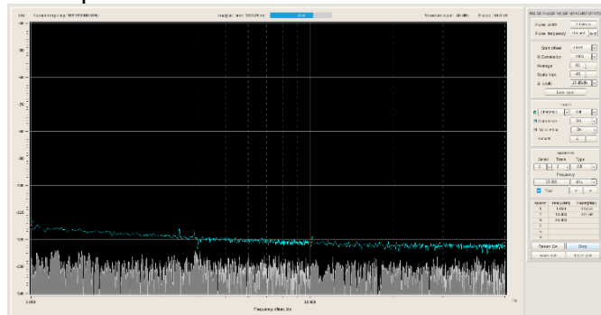
Рис. 7. Результаты измерения фазового шума серийно производимого генератора сигналов на частоте 1 ГГц в режиме импульсной модуляции
