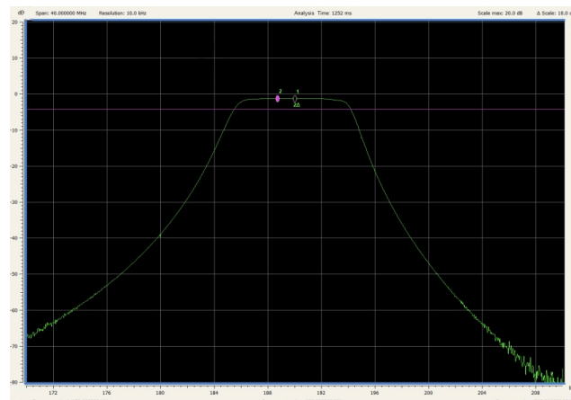
Рис 9. Результат измерения ПП фильтра с использованием встроенного генератора
