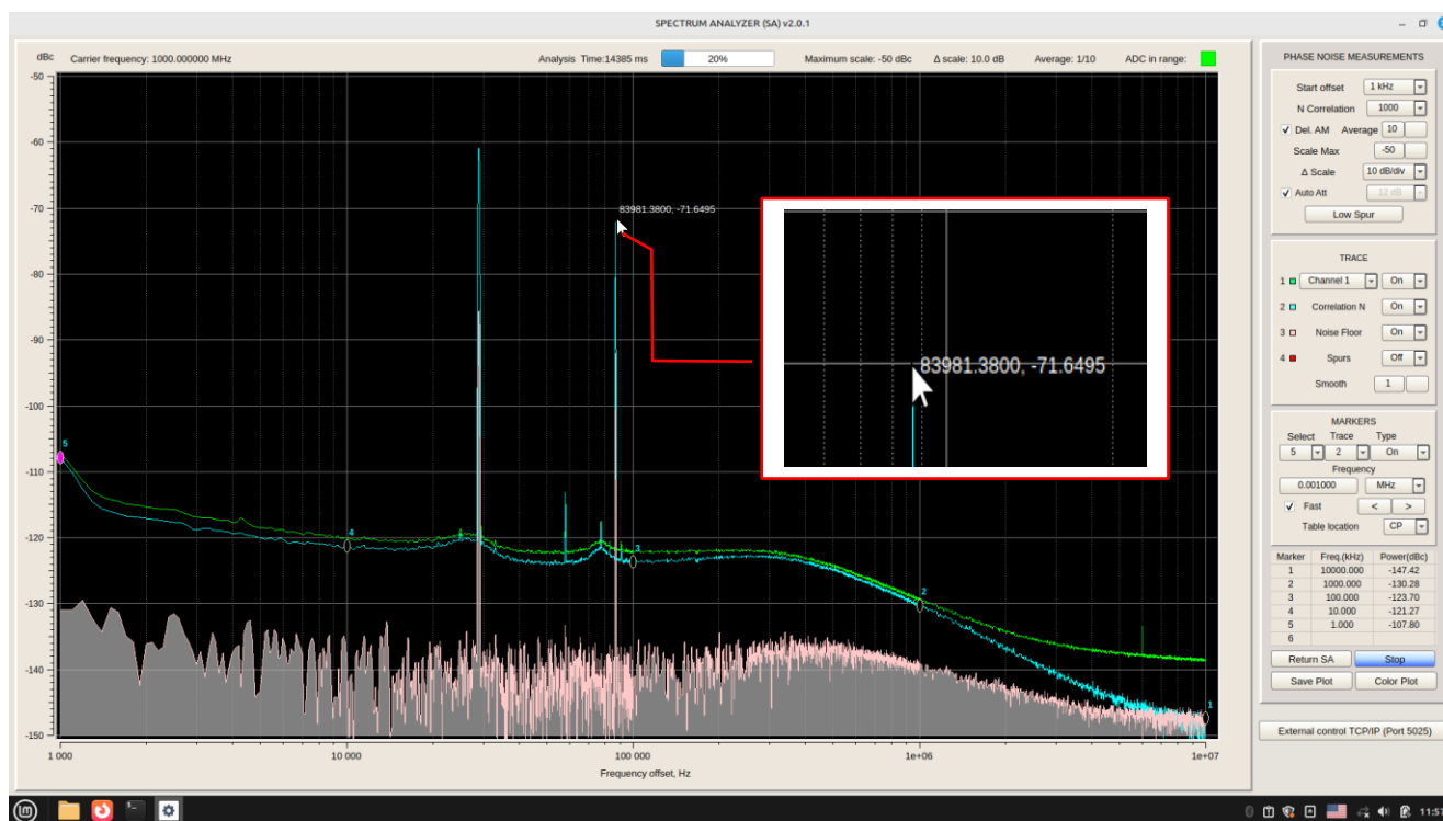
Рис. 1. Режим измерения ФШ с индикацией возможности снятия характеристик с помощью курсора
