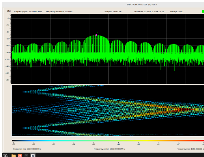
Рис.3. Режим одновременного наблюдения частотной развертки и диаграммы «водопад»
