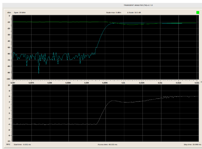
Рис 10. Анализ переходных процессов при изменении частоты генератора на 10 МГц.
