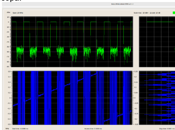
Рис.5. Отображение импульсного сигнала с внутриимпульсной частотной модуляцией
