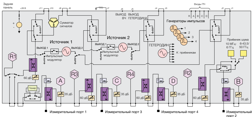
Структурная схема 4-портовых ВАЦ моделей N5244/45B с опцией измерений коэффициента шума 1
