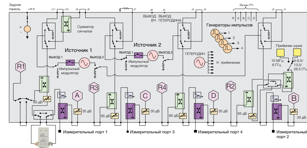
Структурная схема 4-портовых ВАЦ моделей N5241/42/49B с опцией измерений коэффициента шума 1
