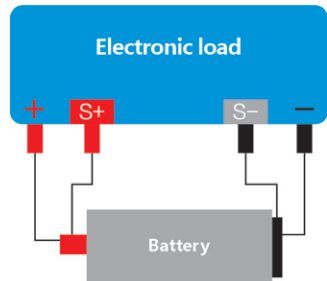
▲ Discharge Wiring
