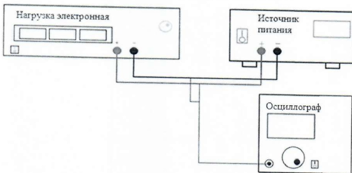
Рисунок 3 – Структурная схема соединения приборов
