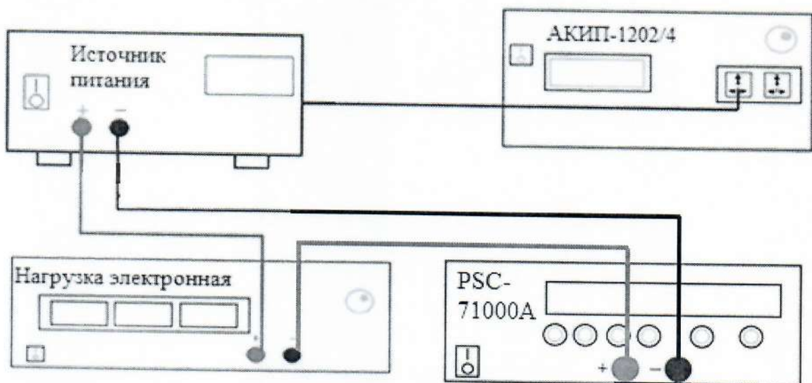
Рисунок 5 – Структурная схема соединения приборов
