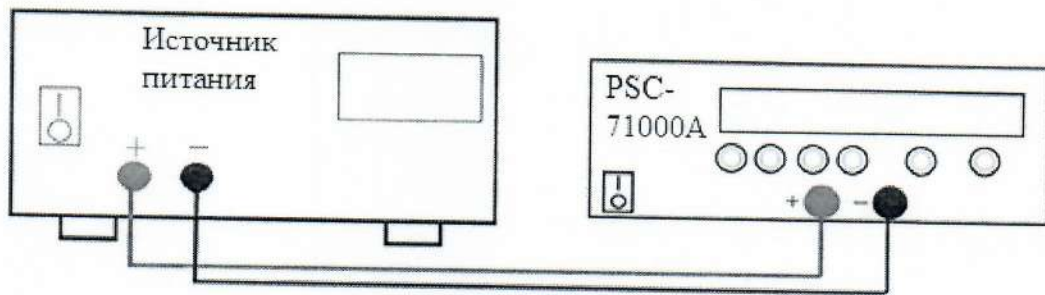
Рисунок 4 – Структурная схема соединения приборов
