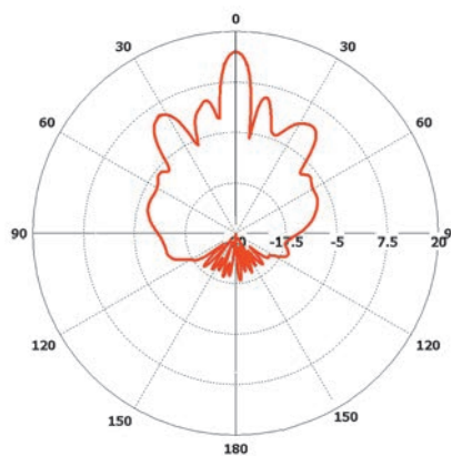
Вертикальная плоскость для порта V
