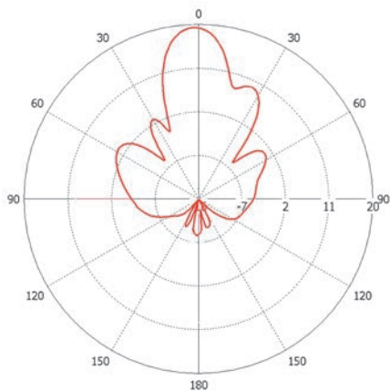
Горизонтальная плоскость
