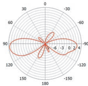
Вертикальная плоскость
