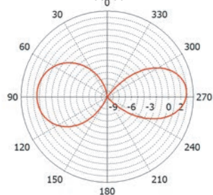
Вертикальная плоскость
