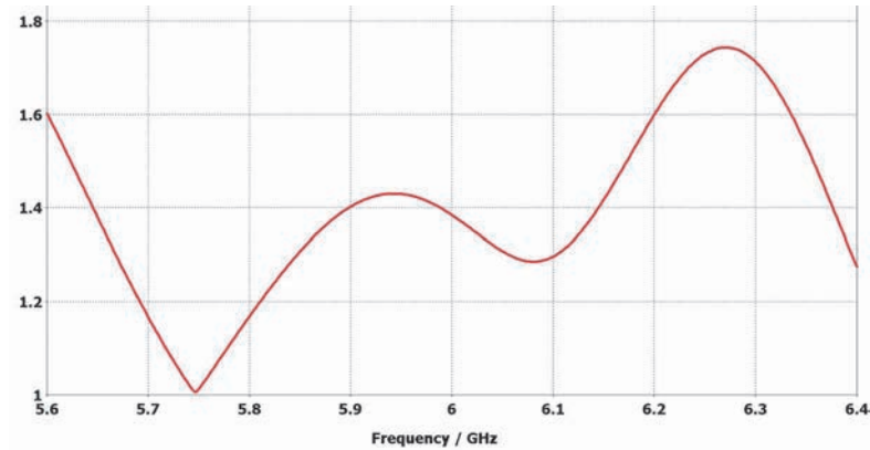
Порт Н
