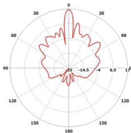
Вертикальная плоскость для порта H
