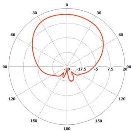
Горизонтальная плоскость для порта V
