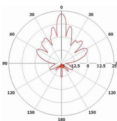
Вертикальная плоскость для порта H
