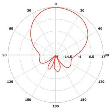
Горизонтальная плоскость для порта H
