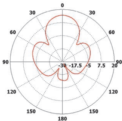
Горизонтальная плоскость
