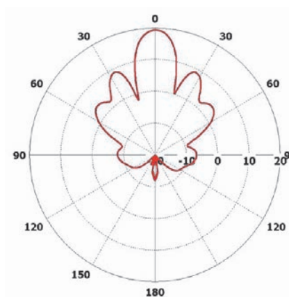
Вертикальная плоскость
