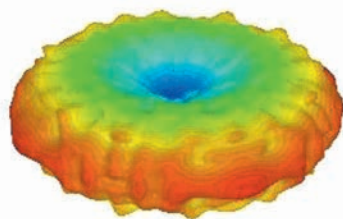
18 ГГц
