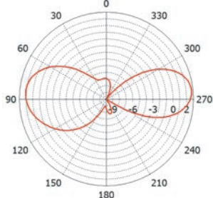
Вертикальная плоскость
