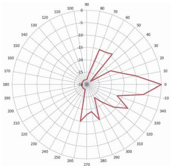
Диаграмма направленности на частоте 1.1 ГГц
