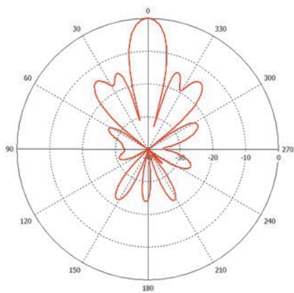
Горизонтальная плоскость
