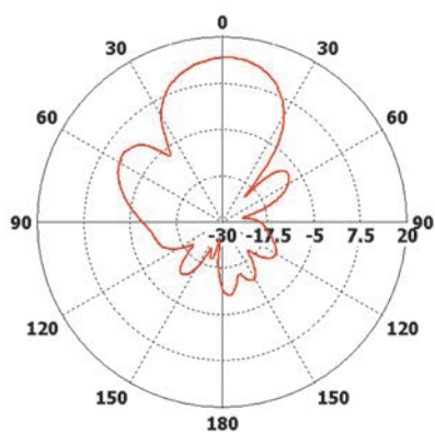
Вертикальная плоскость
