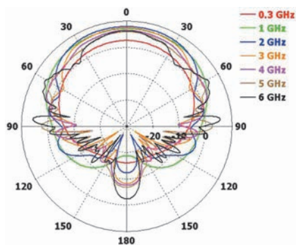
Горизонтальная плоскость
