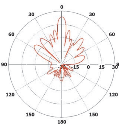
Вертикальная плоскость для порта V
