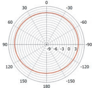
Горизонтальная плоскость
