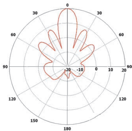
Горизонтальная плоскость
