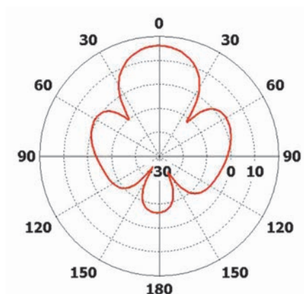
Горизонтальная плоскость
