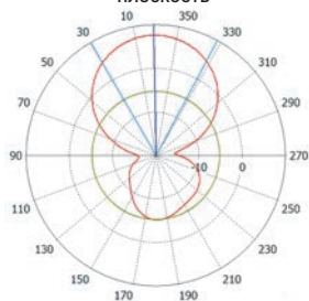
Горизонтальная плоскость
