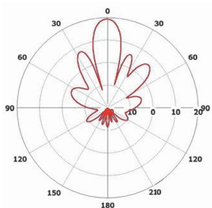
Горизонтальная плоскость
