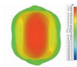
3 ГГц
