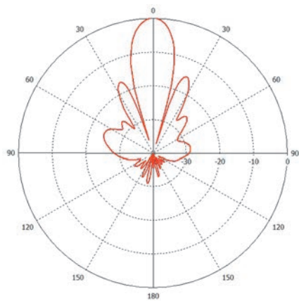
Горизонтальная плоскость
