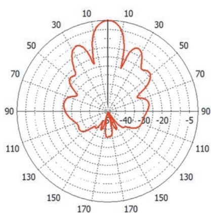
Вертикальная плоскость
