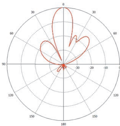
Вертикальная плоскость
