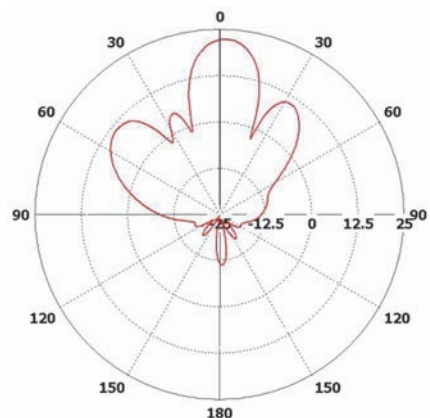
Горизонтальная плоскость для порта H
