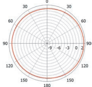
Горизонтальная плоскость
