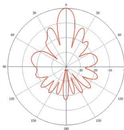
Вертикальная плоскость
