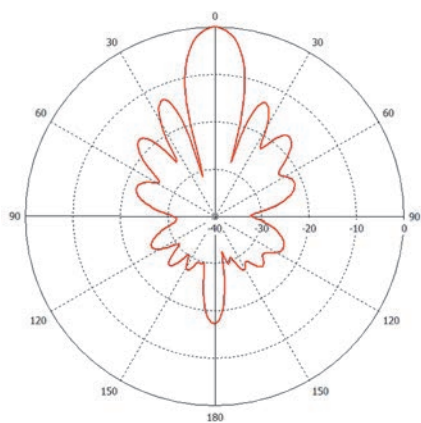
Горизонтальная плоскость
