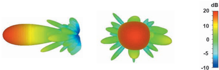
Вертикальная плоскость
