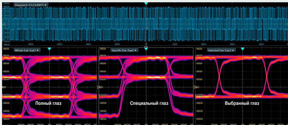
Анализ сигналов АИМ-4: глазковая диаграмма в режимах полного, специального или выбранного глаза
