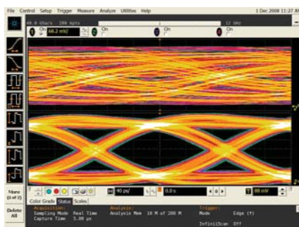
Уменьшение ошибок приёмника посредством открытия полностью закрытых глазков.
