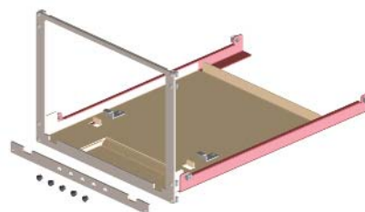
Монтаж осциллографа серии 9000 в стандартную стойку шириной 19 дюймов (487 мм) с помощью опции ICM.
