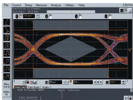
Восстановление встроенных сигналов синхронизации с помощью программы анализа последовательных потоков данных
