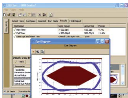
Испытание на соответствие стандартам USB
