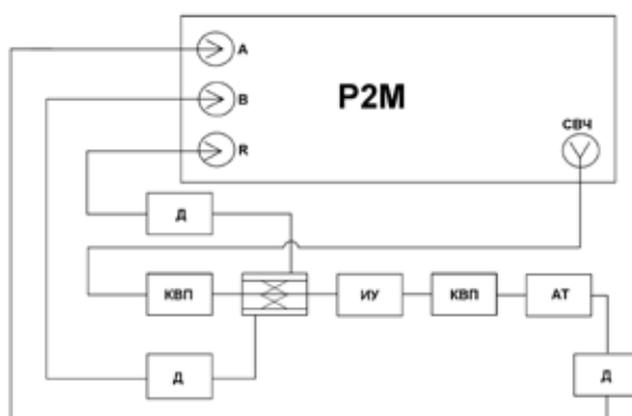
Д — детектор, КВП — коаксиально-волноводный переход, АТ — аттенюатор, ИУ — измеряемое устройство
