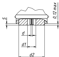
Присоединительные размеры ПКМ2 с приборной стороны
