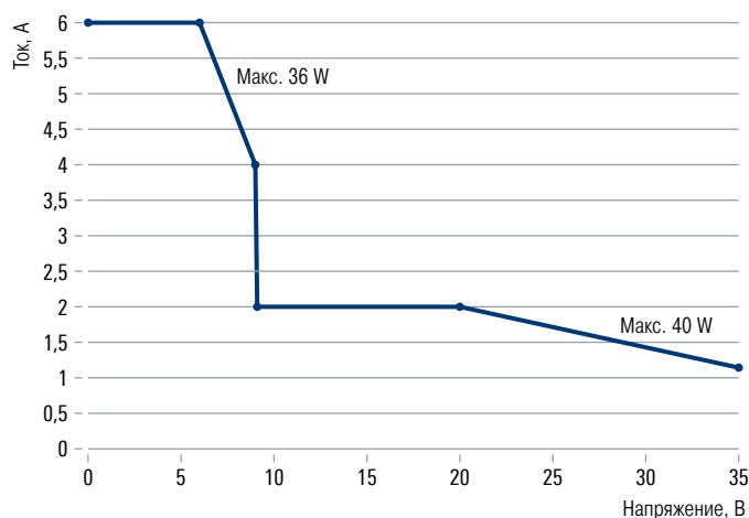
Кривая FlexPower отдельного выхода источника R&S®NGA101/R&S®NGA102
