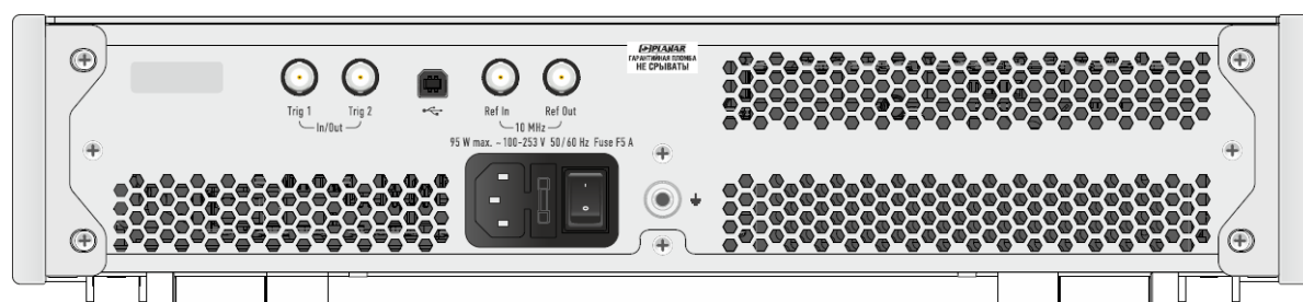
Рисунок 15— Задняя панель
